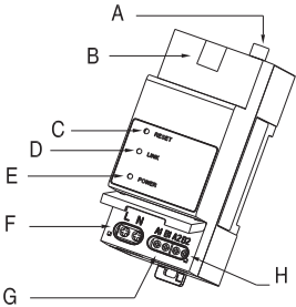
Fig 1: Definición de eSolar SEC-C
