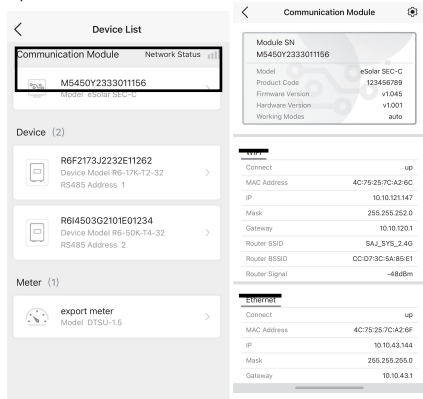
Fig 8: Conexión de la interfaz SEC-C de eSolar
