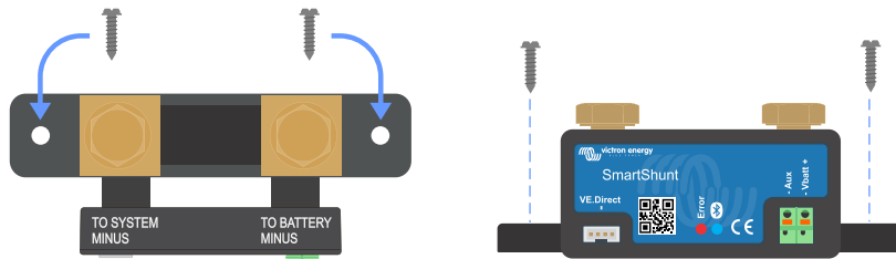
Vista superior del SmartShunt mostrando los orificios de montaje y vista lateral del SmartShunt mostrando el método de montaje.
