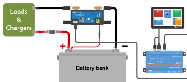
Ejemplo de un monitor de baterías conectado a un dispositivo GX.
